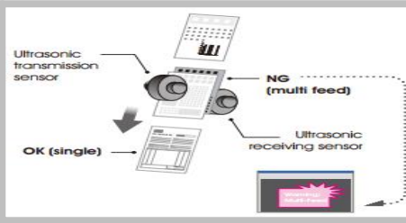
이중급지 감지 Ultrasonic Sensor
